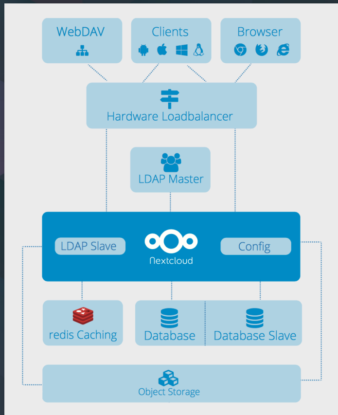
* Nextcloud 服务架构
